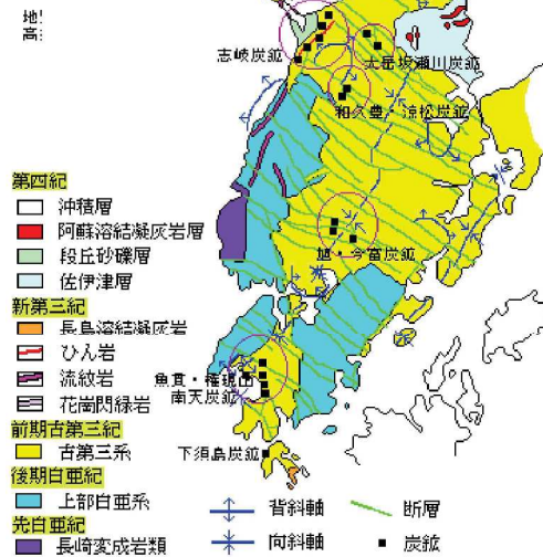
天草炭田地域の地質略図
